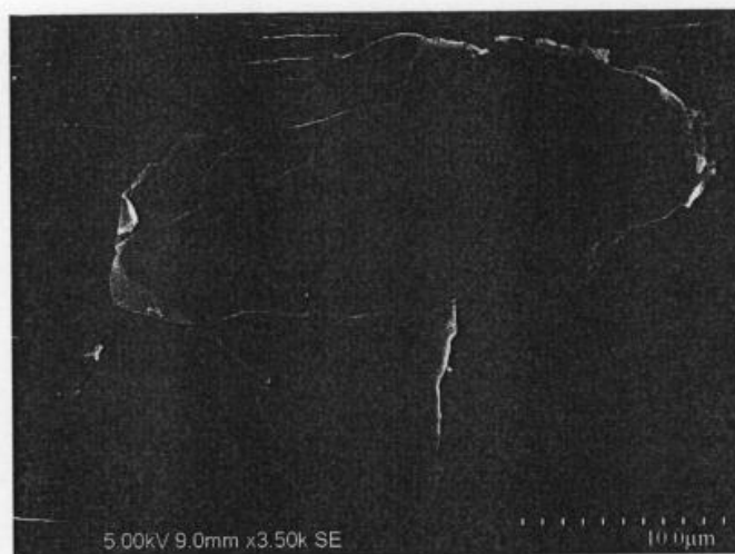
图 C.3 铝粉的扫描电镜形貌图
