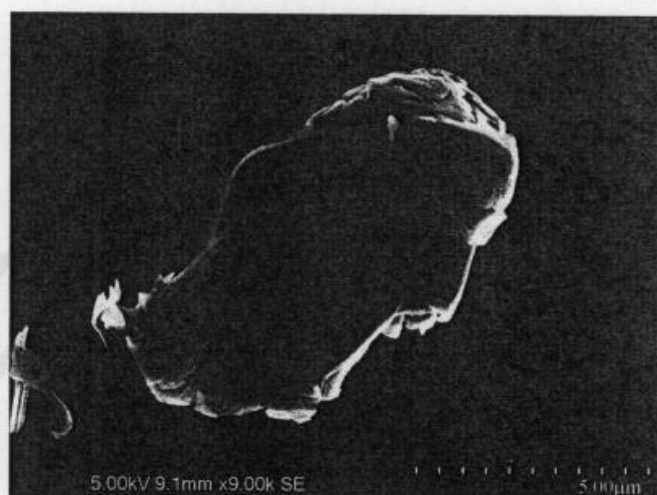
图 C.1 石墨的扫描电镜形貌图
