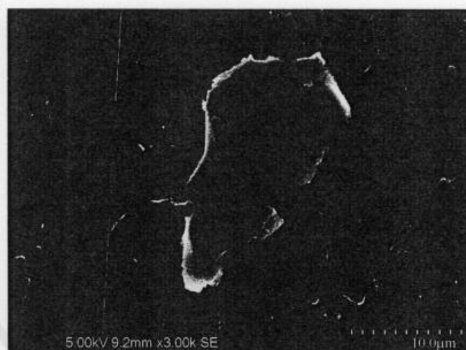
图 C.6 云母的扫描电镜形貌图
